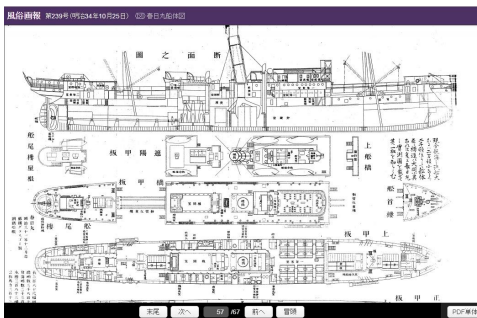
〈図〉春日丸船体図 風俗画報 第 239号 「来客案内郵船図会」(明治 34年10月25日) より
